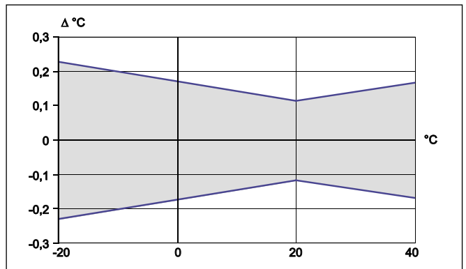
HMP155超过温度范围的测量准确度
